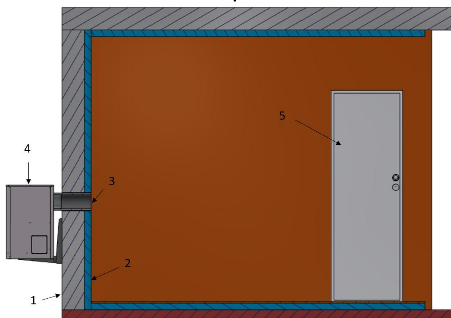
Coupe
